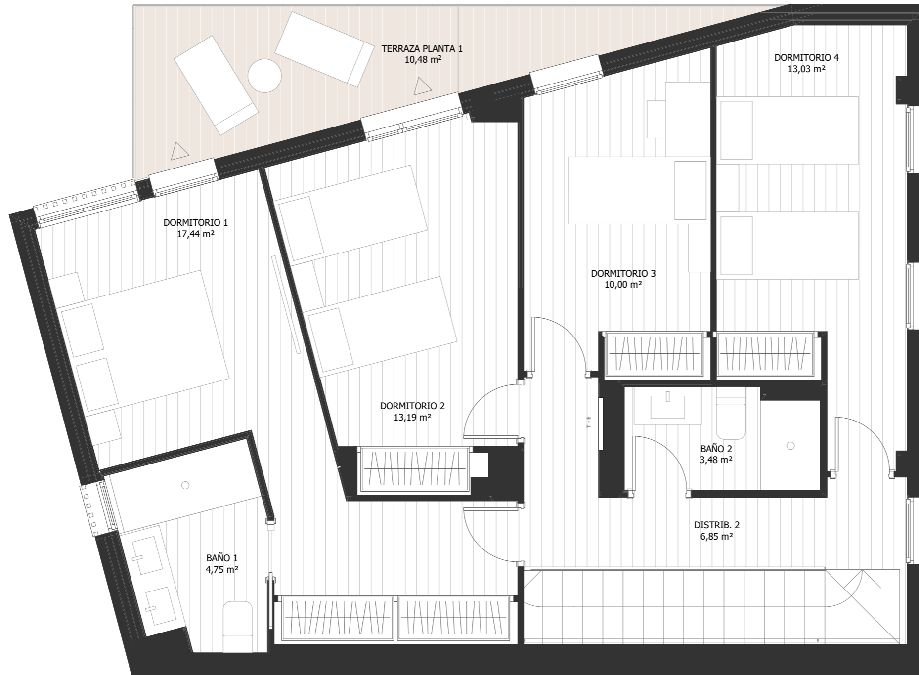
PLANTA PRIMERA
