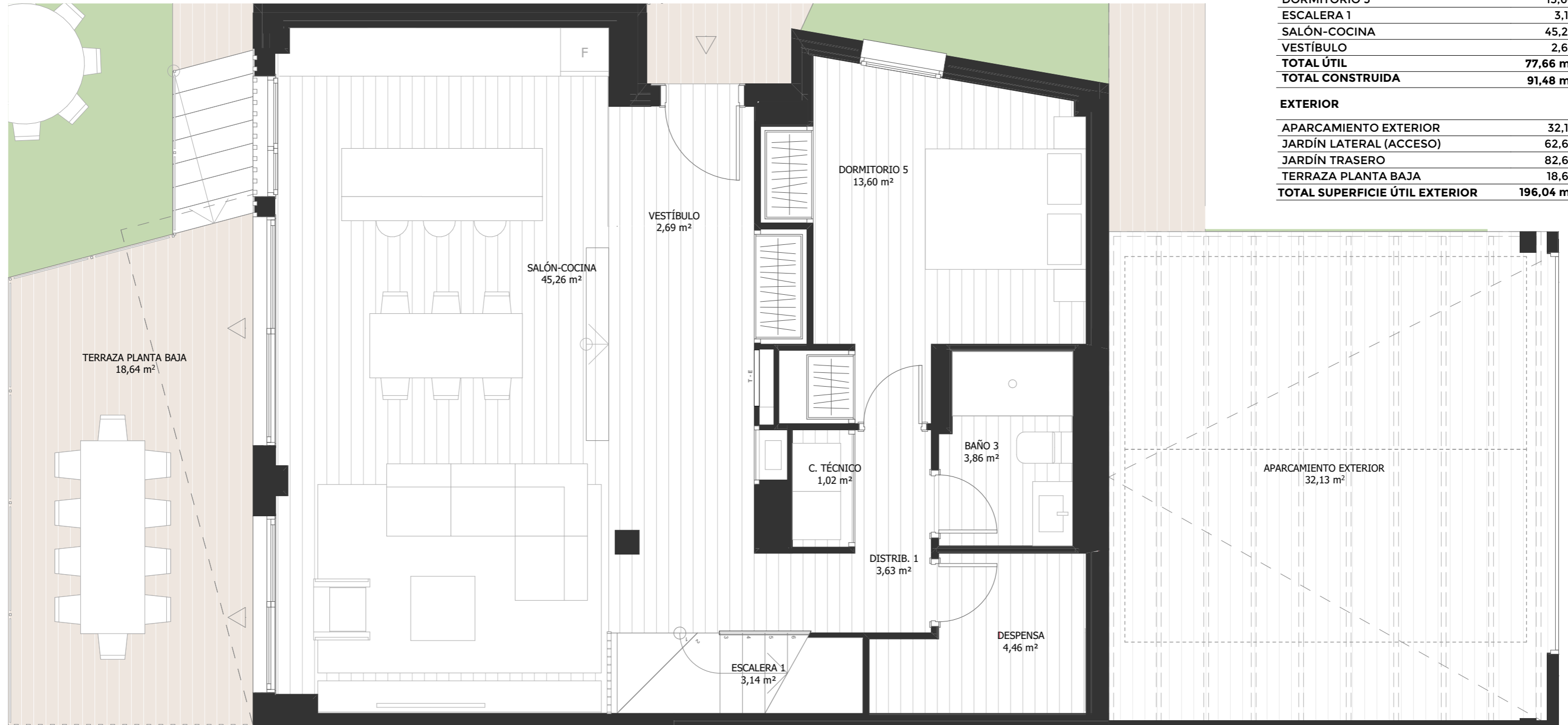
PLANTA BAJA
